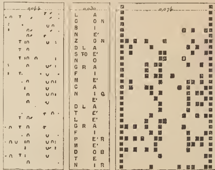
Fig. 4 Fig. 5 Fig. 6 Impresiones y tira de papel perforado del telégrafo taquigráfico
